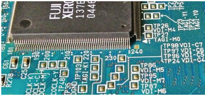
Resim 1. Bir elektronik kontrol kartı üzerindeki TP noktalarından bazıları
